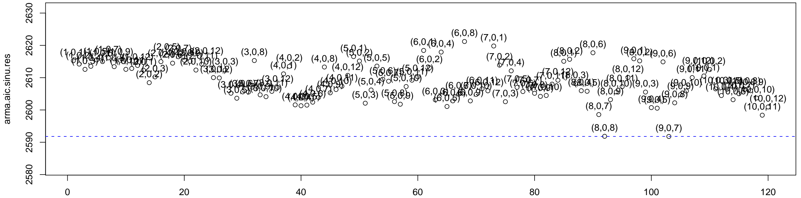
ARIMA(p=[1:10],0,q=[1:12]) aic Values
