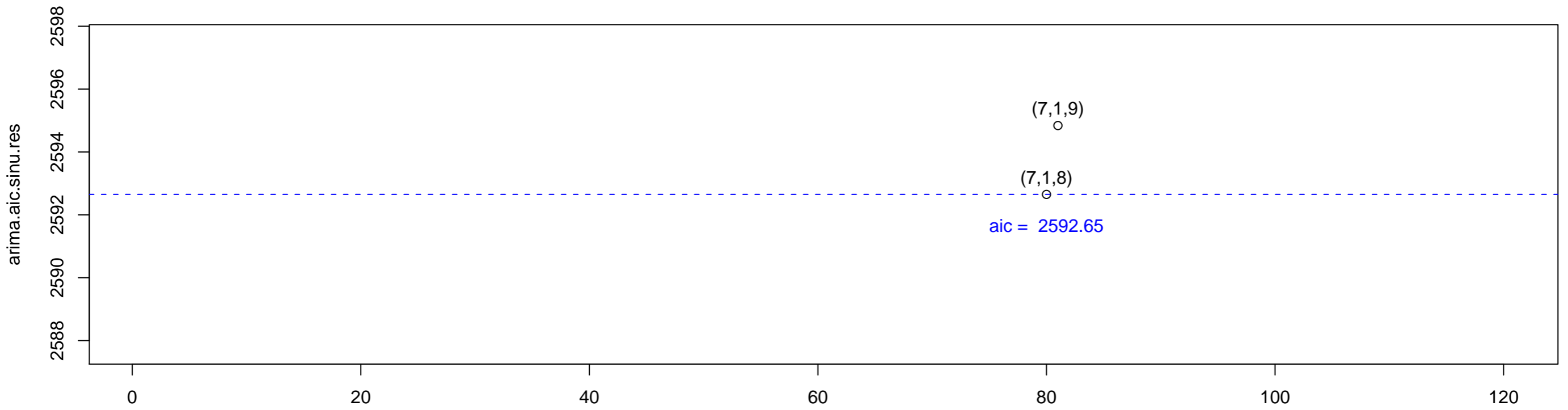
ARIMA(p=[1:10],1,q=[1:12]) aic Values
