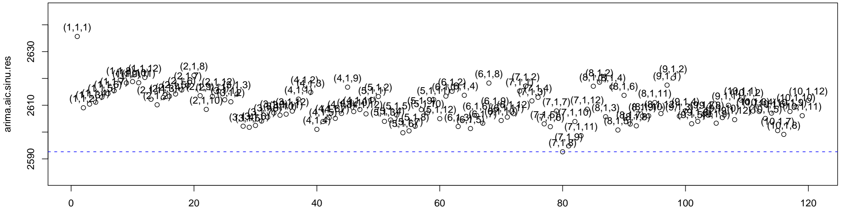
ARIMA(p=[1:10],1,q=[1:12]) aic Values
